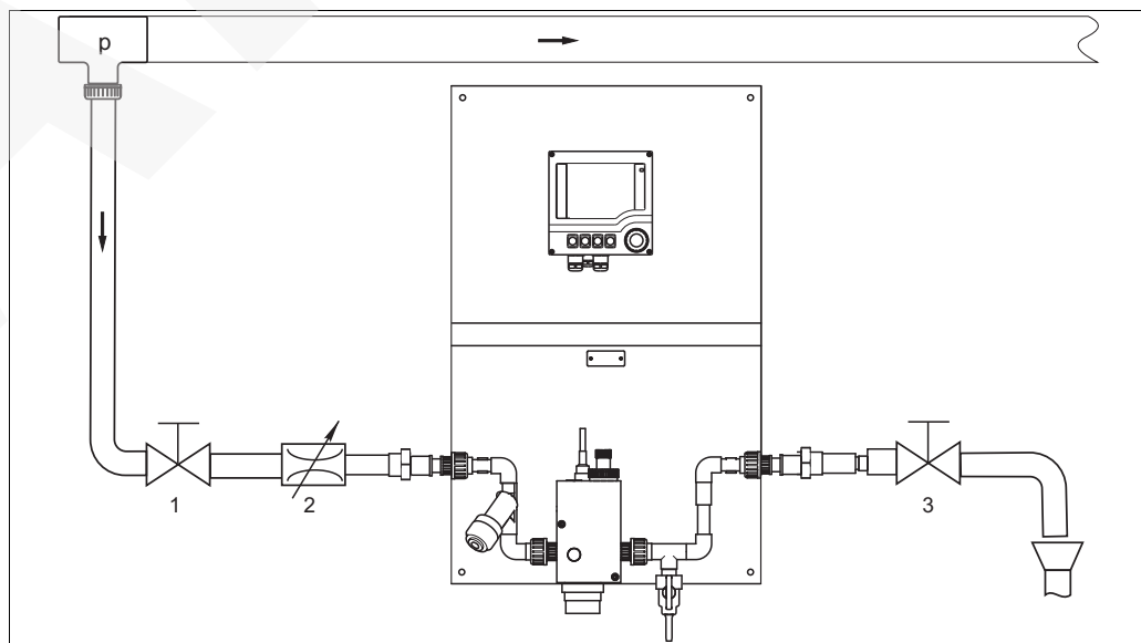
在带开放式出水口的管道中安装的安装示意图
